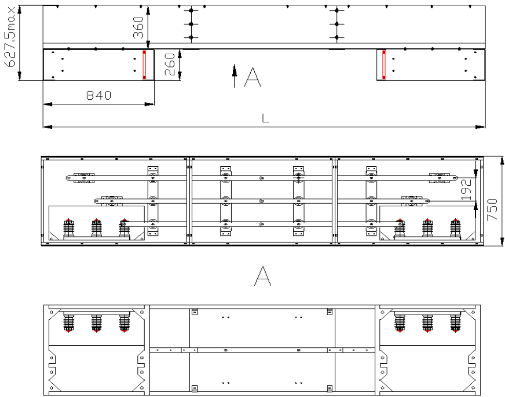
Рисунок 3 – Шинный мост
