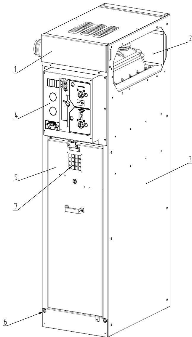
Рисунок 1 – Ячейка КСО
