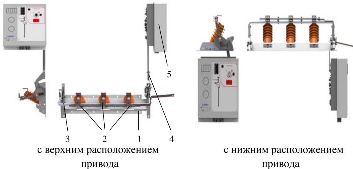
Рисунок 4 – Заземлитель SL
